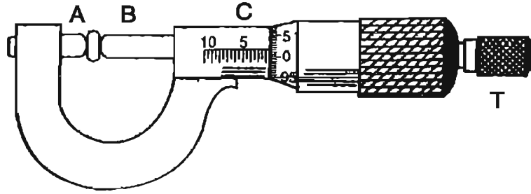
চিত্র ২.৩ স্ক্রু গজ
