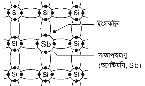
চিত্র : ২২.৩ n-টাইপ অর্ধপরিবাহী
