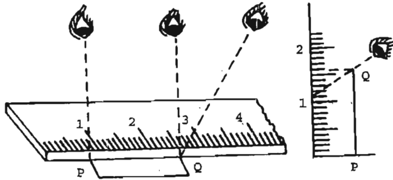
চিত্র-১ : স্কেল ব্যবহারের ভুল পদ্ধতি
