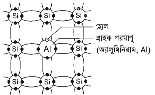
চিত্র : ২৩.২ p-টাইপ অর্ধপরিবাহী
