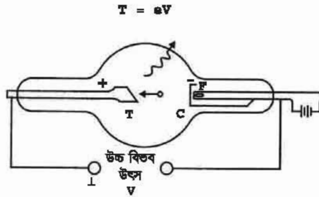
চিত্র : ২৪.১ একটি এক্সরে টিউবের প্রয়োজনীয় অংশ
