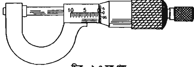
চিত্র : ২.৪ স্ক্রু গজ
